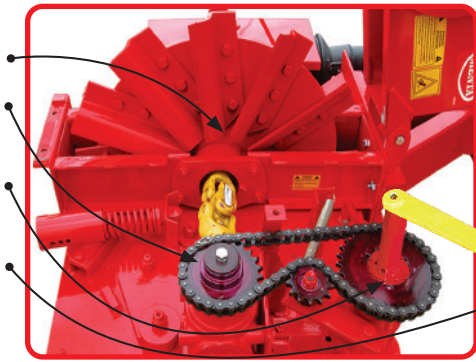
• Afiador rotativo das facas. • Afiador rotativo de cuchillas.
