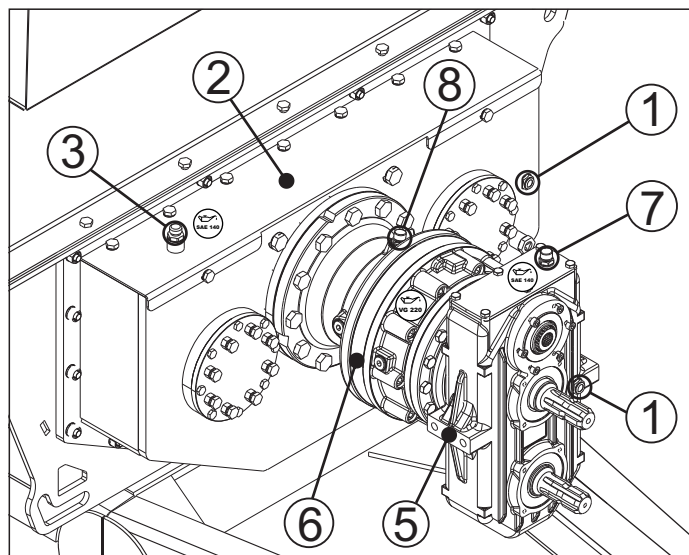
Fig. 19 - Caixa de Engrenagen e Planetário
